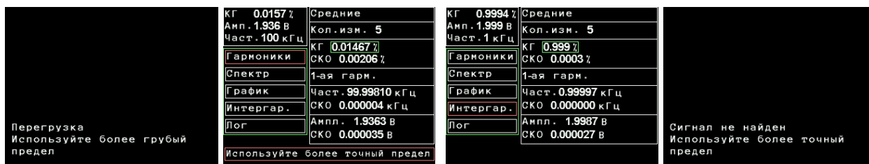
Рисунок 2.9. Разные сообщения при использовании ручного выбора предела измерения. Слева направо – перегрузка, неполное использование динамического диапазона АЦП, корректный выбор предела измерения, невозможность определения параметров сигнала
