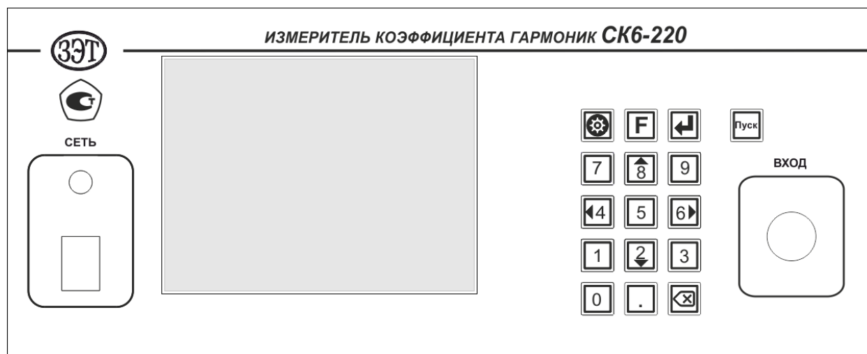
Рисунок 2.1. Внешний вид передней панели измерителя коэффициента гармоник СК6-220
