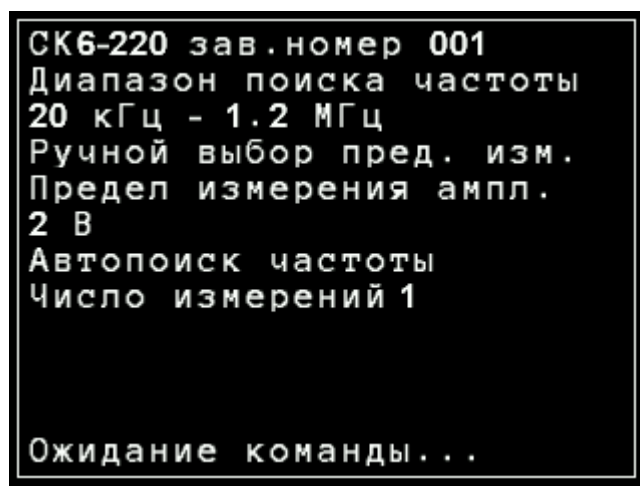
Рисунок 2.2. Главное окно измерителя коэффициента гармоник СК6-220
