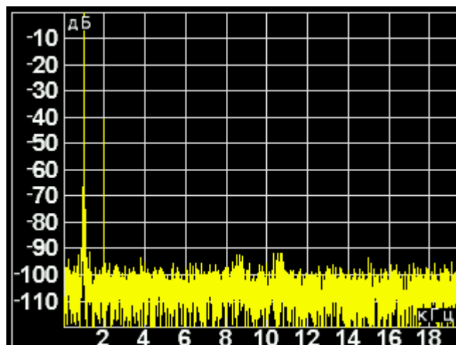
Рисунок 2.16 Спектр измеряемого сигнала
