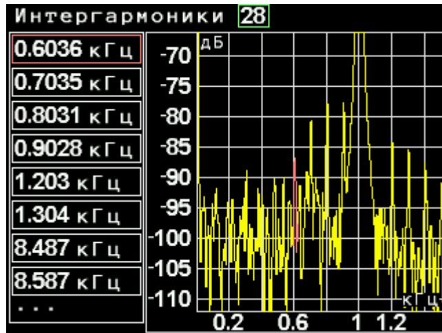
Рисунок 2.19. Визуализация части спектра с текущей выбранной интергармоникой
