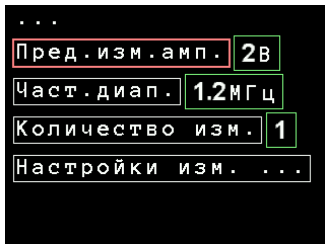
Рисунок 2.6. Подменю «Настройки ...»
